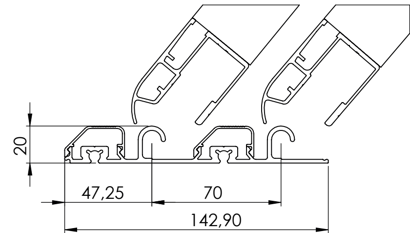
DETAIL A MĚŘITKO 1 : 2
